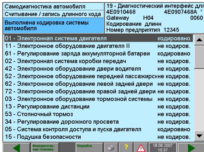
Рис. 6-3 Окно «Выбор систем автомобиля для кодировки»
