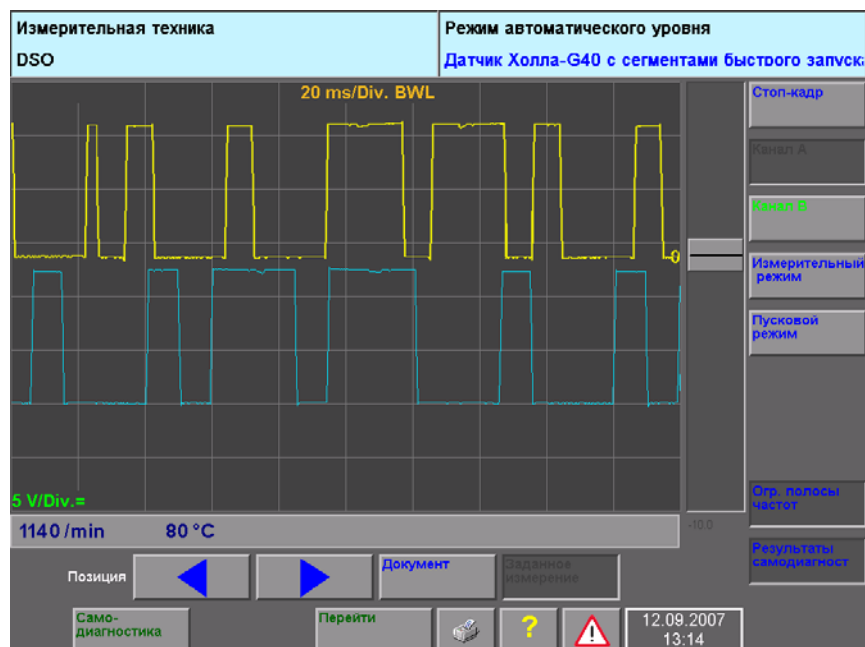
Рис. 5-24 Окно «DSO» с примерами индикации значений OBD
