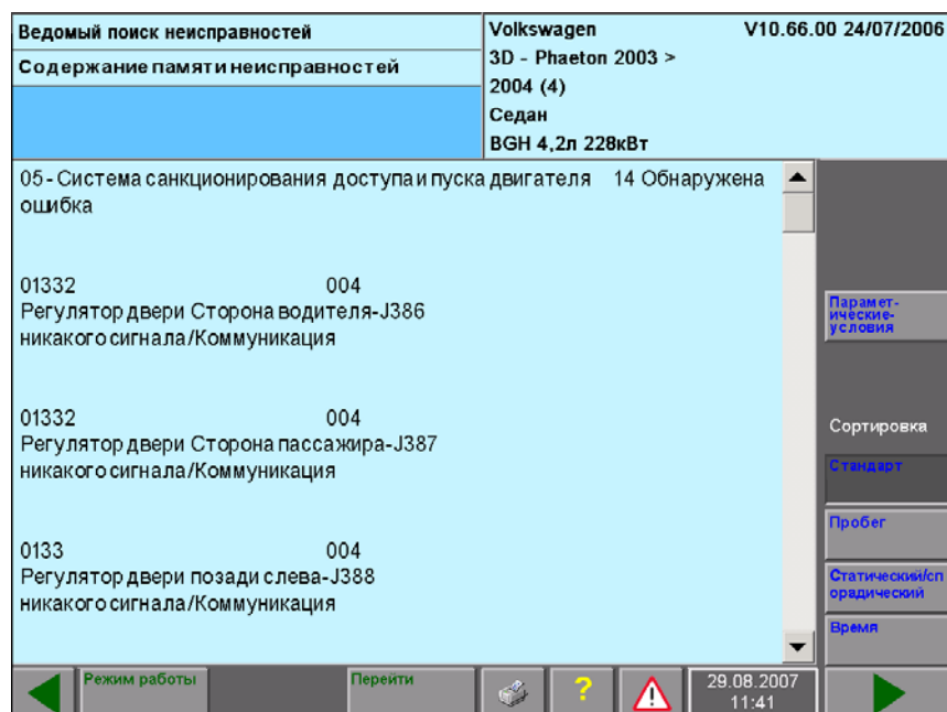
Рис. 6-9 Окно «Содержание памяти неисправностей», сортировка «Стандарт»
