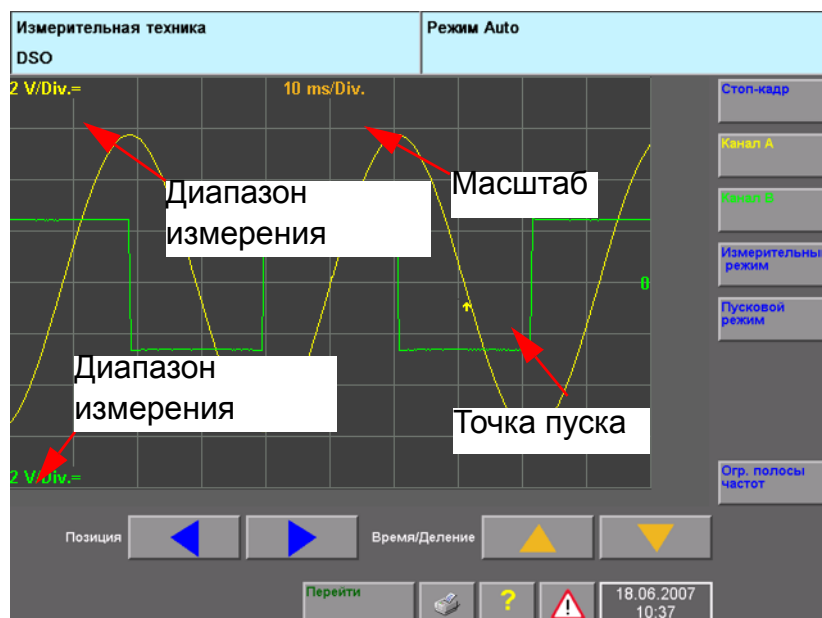
Рис. 5-12 Окно «DSO», базовая установка
