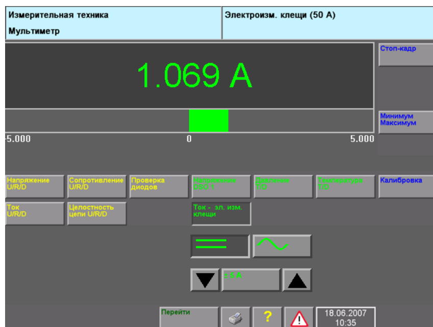
Рис. 5-5 Окно «Мультиметр», измерение силы тока с помощью токоизмерительных клещей на 50 А
