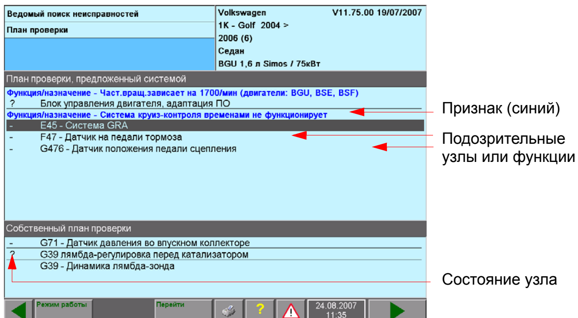
Рис. 6-25 Системный и собственный план проверки с несколькими подозрительными узлами
