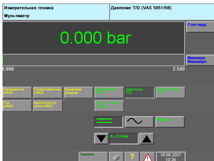
Рис. 5-10 Окно «Давление T/D»
