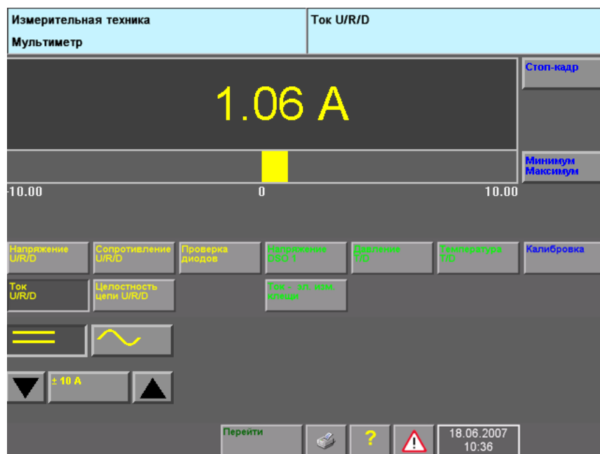
Рис. 5-4 Окно «Мультиметр», измерение силы тока
